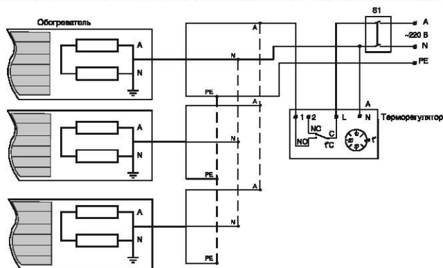
Рис. 1. Обогреватель ВИН-АР-0.8; ВИН-АР-1.0; ВИН-АР-2.0
